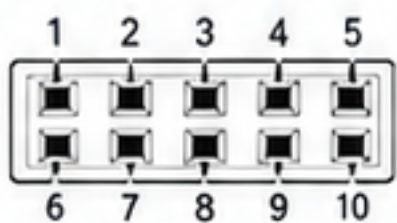
پین‌های سوکت مادگی
