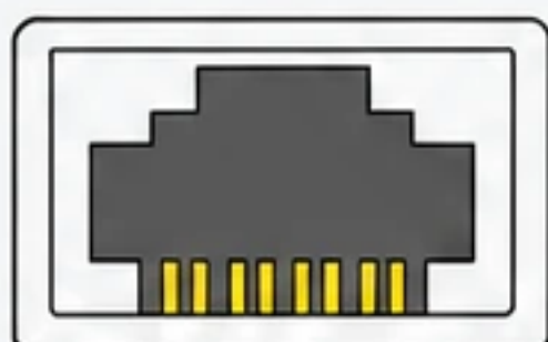
پین‌های سوکت
