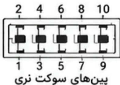
سوکت کابل فلت 2x5 نری
