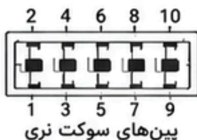
سوکت کابل فلت 2x5 نری
